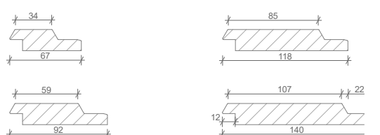
profil DF BUER
