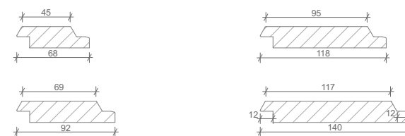
profil DF FAS
